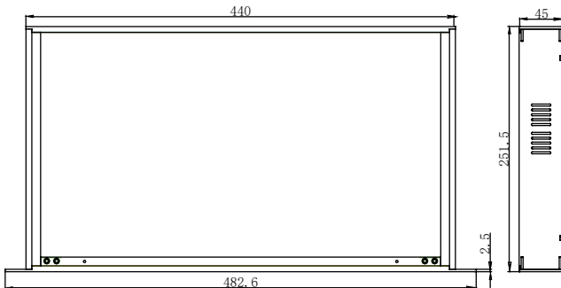
VX4 's dimension (Unit:mm)
